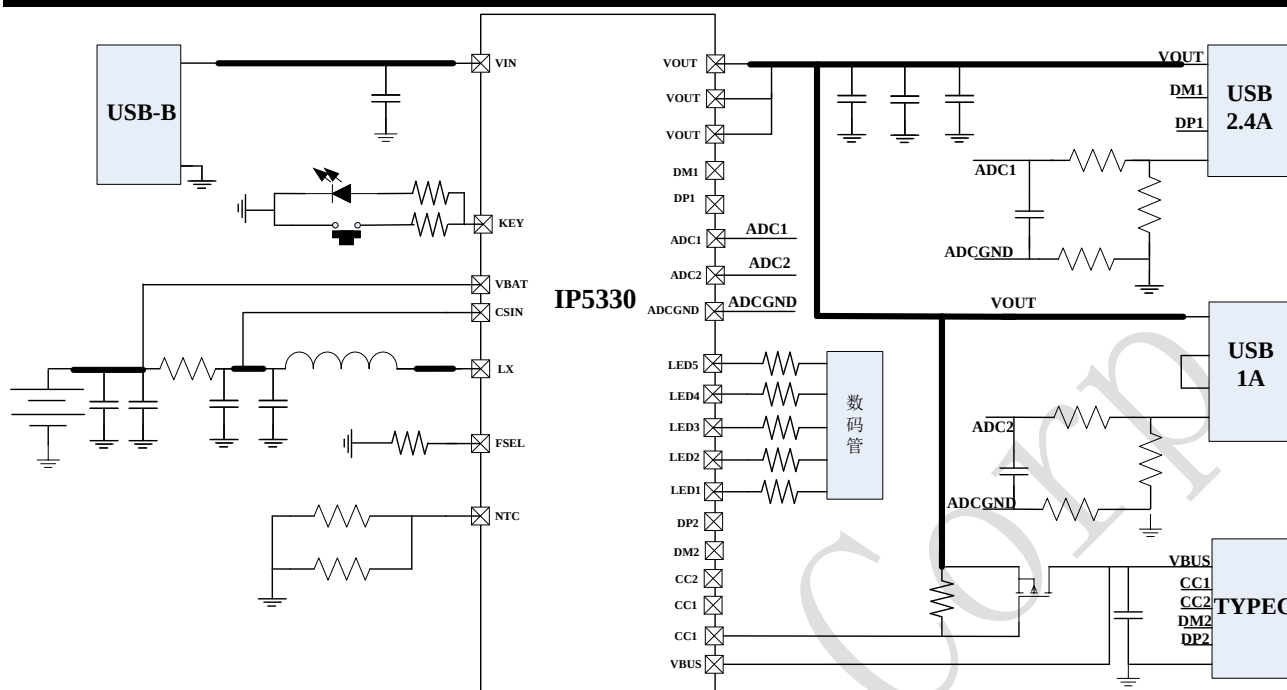
图 1 IP5330 简化应用原理图(数码管显示电量)
